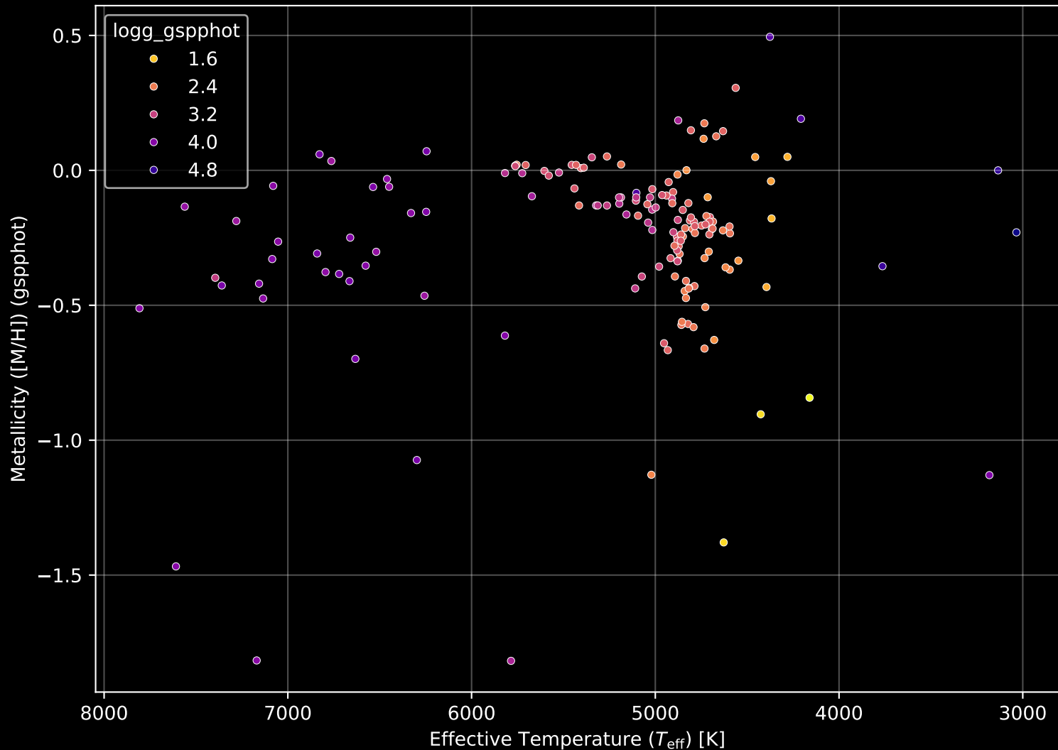
APOGEE DR17 Field: [135+30] Stellar Population Parameters (n= 159)
